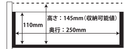
側面図
